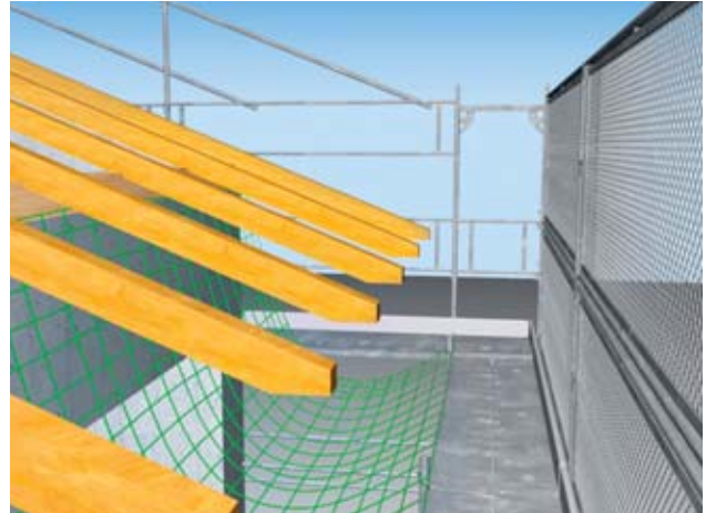
Bild 12 Lösung mit Auffangnetz im Dachvorsprung
