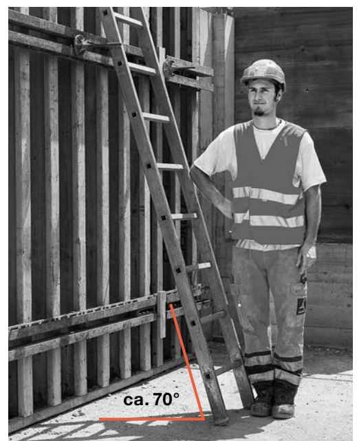
Bild 6: Überprüfen des Anstellwinkels von ca. 70° mit der Ellbogenprobe
